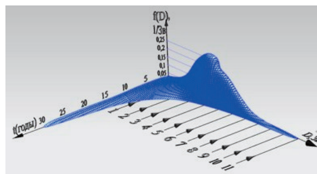
Рис. 4. Фронтальный вид воксель-модели плотности вероятности f(D) выхода стохастических и детерминированных эффектов в зависимости от дозы D (построена по данным табл. 3 и рис. 3)
