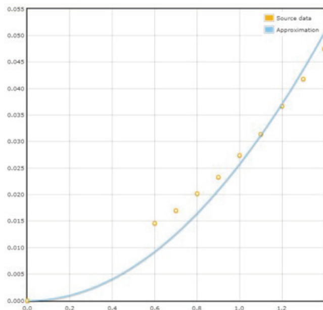
Рис. 2. Стыковка формул (8) и (2), (3) в точке D = 1,1 Зв
