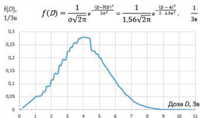
Рис. 3. Плотность вероятности f(D) (формула (1)) выхода стохастических и детерминированных эффектов в диапазоне доз от 0 до 11 Зв с шагом 0,1 Зв (по данным табл. 3)
